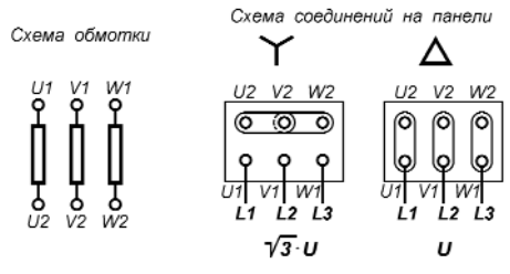
Рисунок 7.1 для односкоростных двигателей с соединением в звезду (Y), в треугольник (Δ) или переключаемых: звезда - треугольник (Y/Δ).
