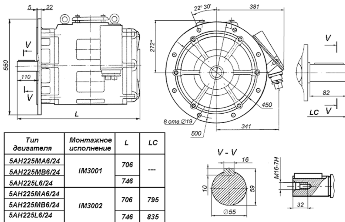
Габаритные, установочные и присоединительные размеры двигателя 5AH225...НЛБ. Монтажное исполнение IM3001, IM3002
