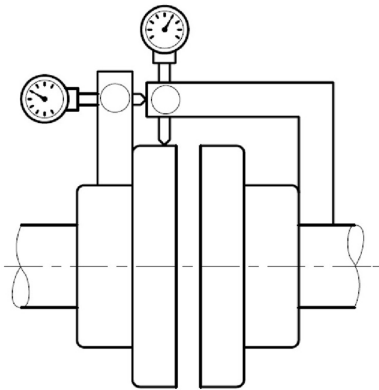
Рис. 3 Схема комбинированного измерения аксиальной и радиальной несоосностей
