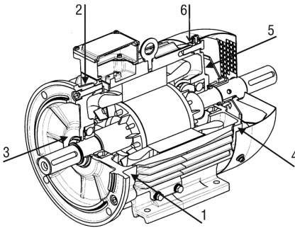
Рис. 1 Точки измерения вибрации
