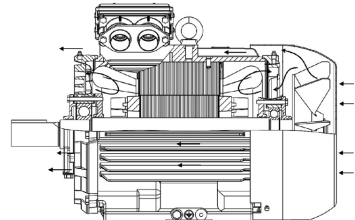
б) с комбинированной системой вентиляции
